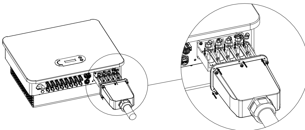
Figura 19 - Conexión de los cables de salida CA (1)
