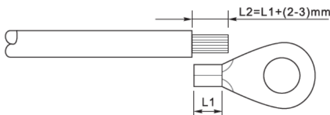
Figura 10 - Preparación del cable de tierra (1)
