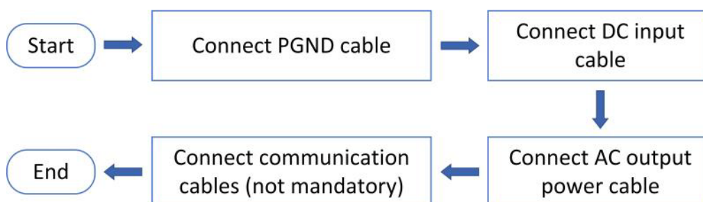
Figura 9 - Fases para la conexión de los cables
