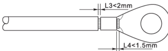
Figura 11 - Preparación del cable de tierra (2)
