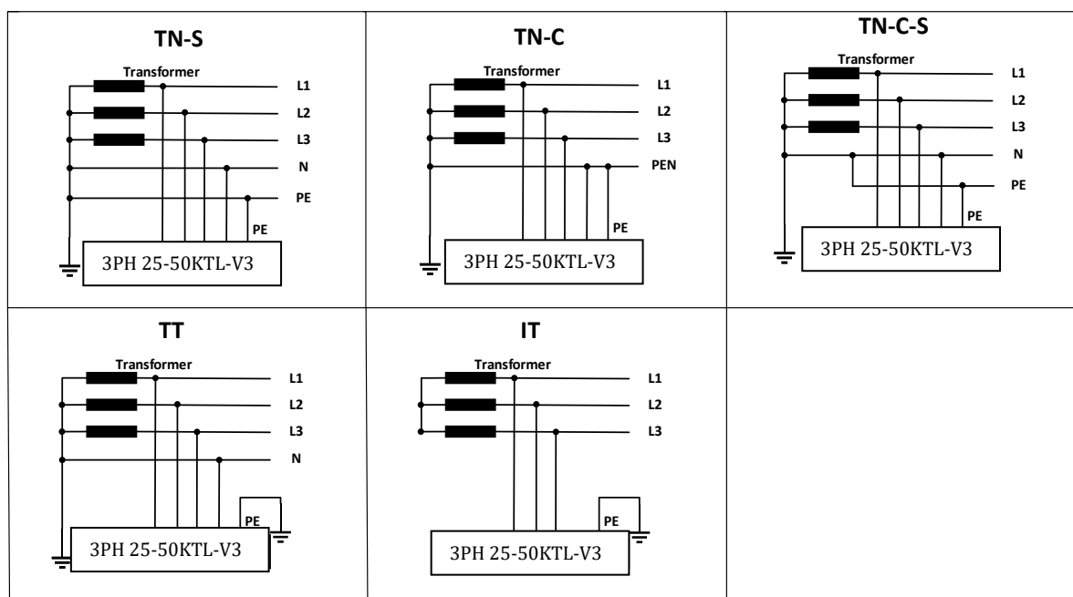
Figura 3 - Esquemas eléctricos de los tipos de red en las que se pueden instalar los inversores 3PH 25KTL-50KTL-V3
