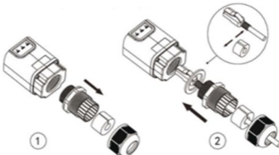
Figura 67 - Introducción del cable de red en el dispositivo
