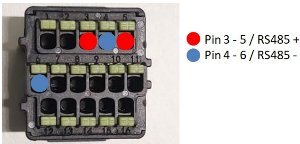
Figura 25 - Conexión de la línea serie mediante conector de comunicación para 3PH HYD5000-HYD20000-ZSS
