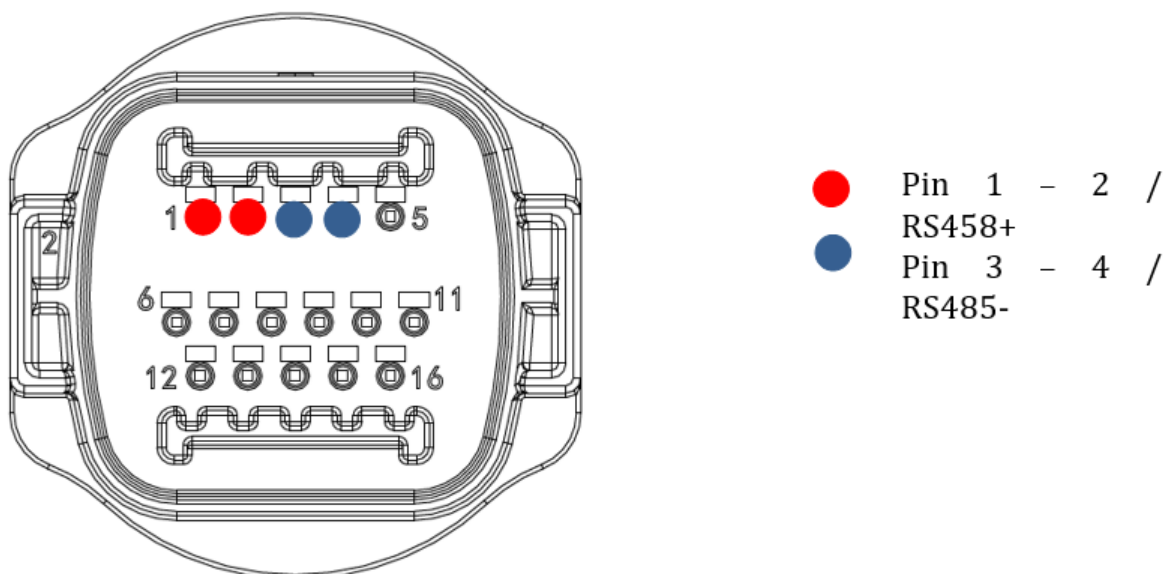
Figura 24 - Conexión de la línea serie mediante conector de comunicación para 1PH 3000-6000 TLM-V3
