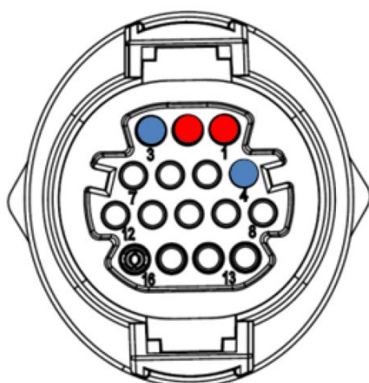
Figura 23 - Conexión de la línea serie mediante conector de comunicación para 3PH HYD5000-HYD20000-ZSS
