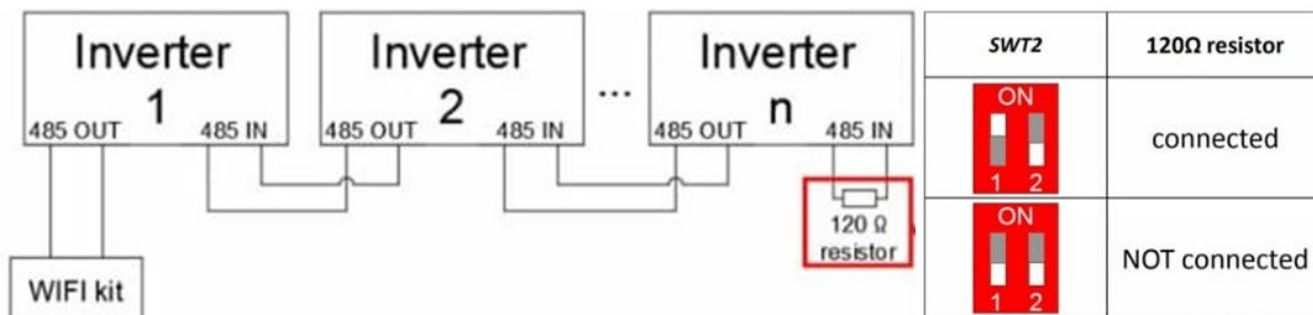
Figura 86- Posición de los interruptores dip para conectar la resistencia de aislamiento
