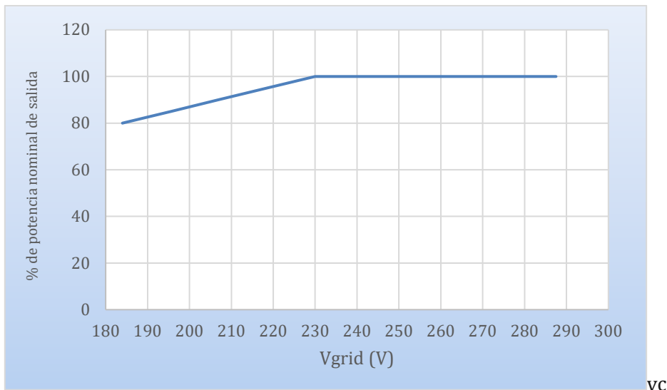
Figura 11 - Relación entre potencia nominal y tensión de red
