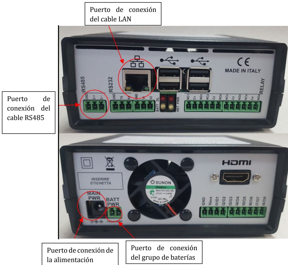
Figura 105 Panel posterior del datalogger
