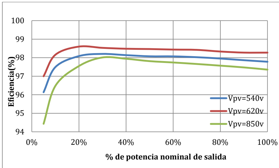
Figura 10 - Curva de eficiencia energética (por ejemplo 50 KW)
