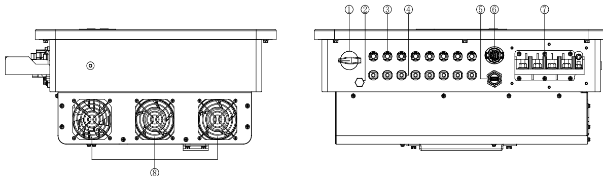
Figura 7- Vista del inversor desde abajo
