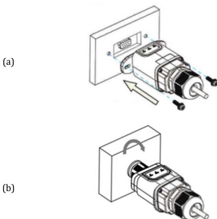
Figura 68 - Introducción y fijación del adaptador Ethernet
