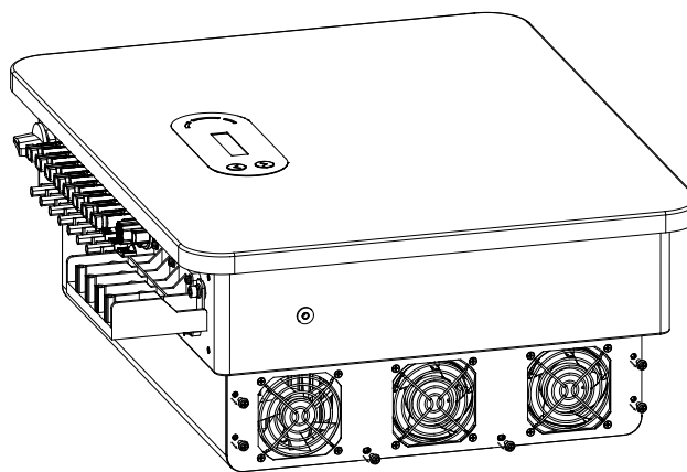
Figura 40 - Retirada de los cuatro tornillos de la placa de base del ventilador
