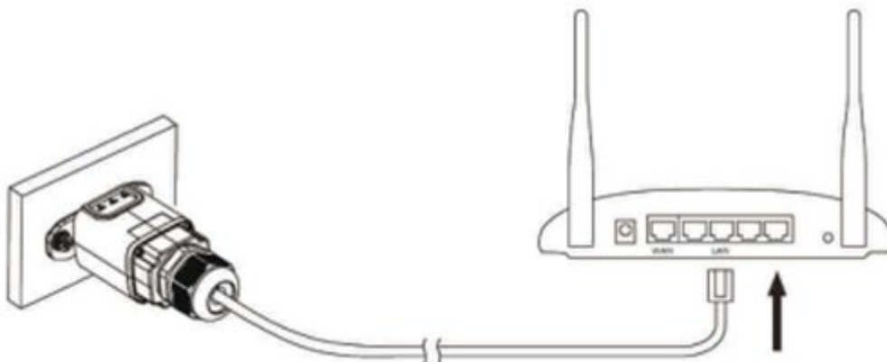
Figura 69 - Conexión del cable de red al módem
