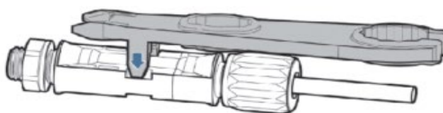
Figura 17 – Extracción del conector CC
