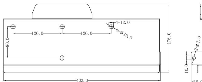
Figura 6 - Medidas del soporte
