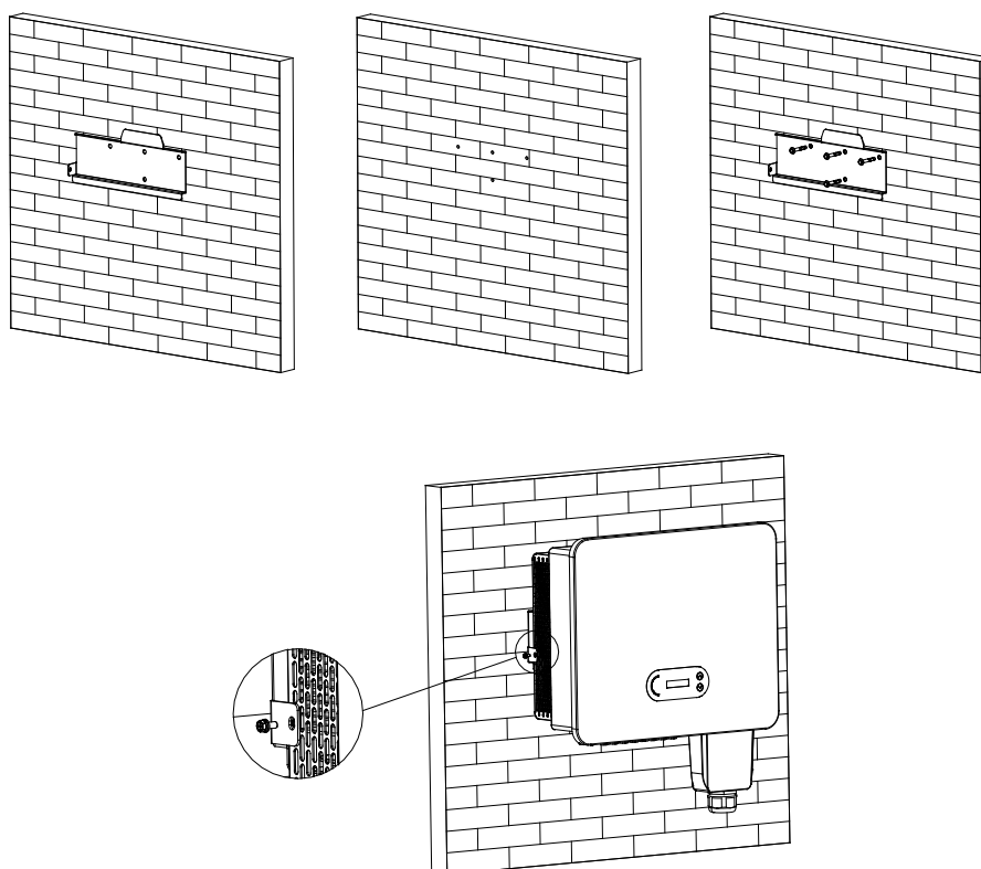
Figura 8 - Fases para el montaje del inversor en la pared
