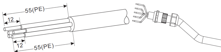
Figura 20 - Conexión de los cables de salida CA (2)
