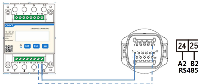
Figura 4 – Posición de los conectores RS485 en inversor
