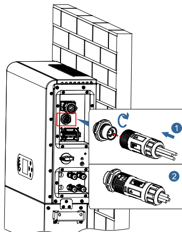
Figura 31 - Conexión EPS
