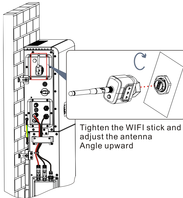
Figura 25 - Conexión WIFI/4G
