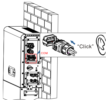
Figura 42 - Conexión COM
