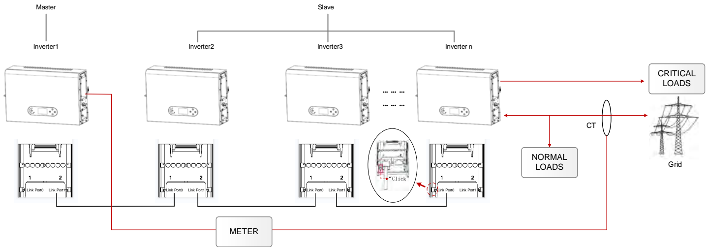
Figura 53- Diagrama del sistema paralelo
