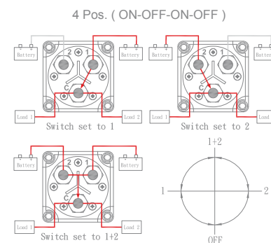
ELE071 4 Posiciones (OFF-BAT1-AMBOS-BAT2)
