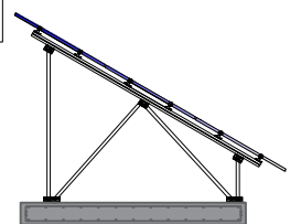
ZAPATA DESCENTRADA
