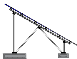
ZAPATA AISLADA
