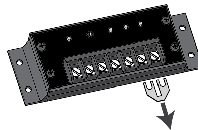
Figura 2a. Extracción del puente de selección de batería.
