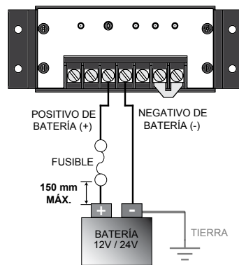
Figura 5. Conexiones de batería
