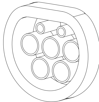
CEI 62196-2 Type 2
