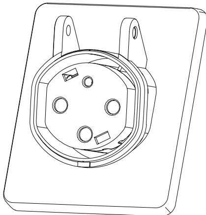
CEI 62196-2 Type 3A
